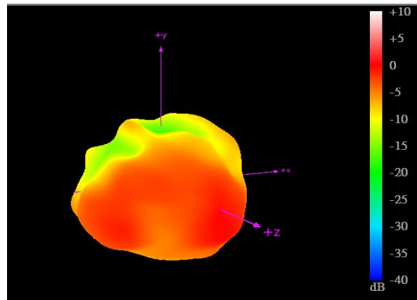
2170MHz
