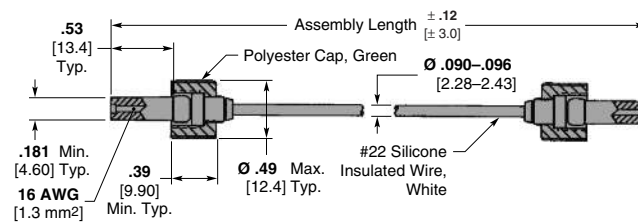
Part Number 449578
