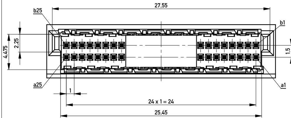
Leiterplatten-Layout Vorschlag / PCB-layout proposal
