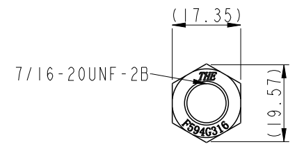
Nut
