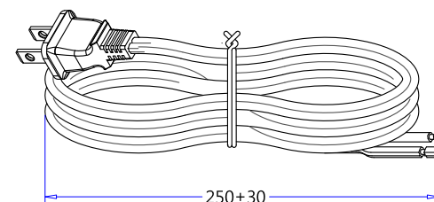
B-C3 扎線圖示 (Tied Loop Hank Detail)
