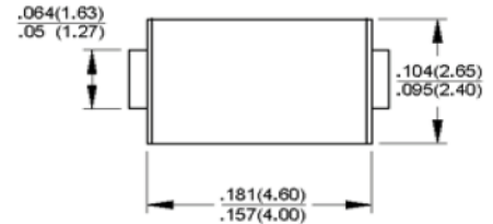
DO-214AC (SMA)
