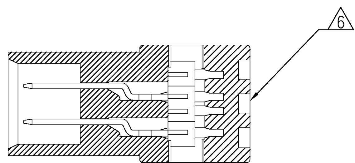
SEC. A-A
