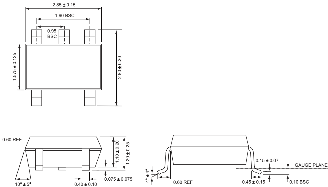
SOT23-5
