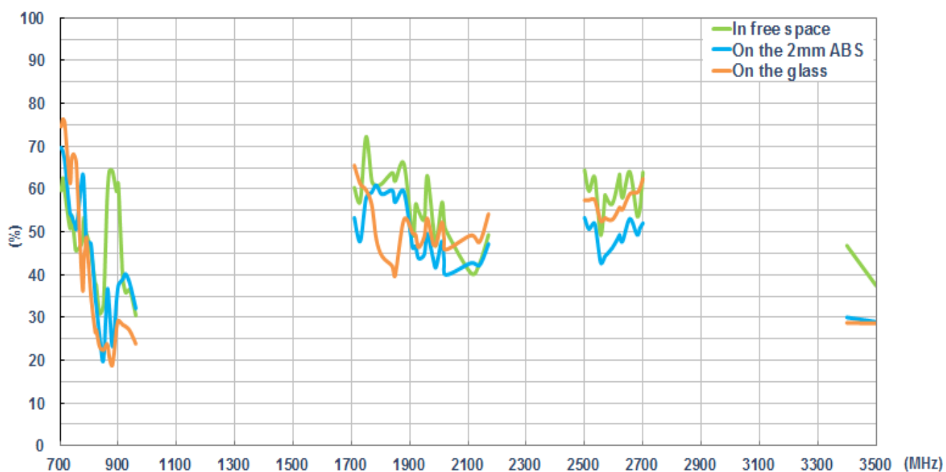
MIMO 2
