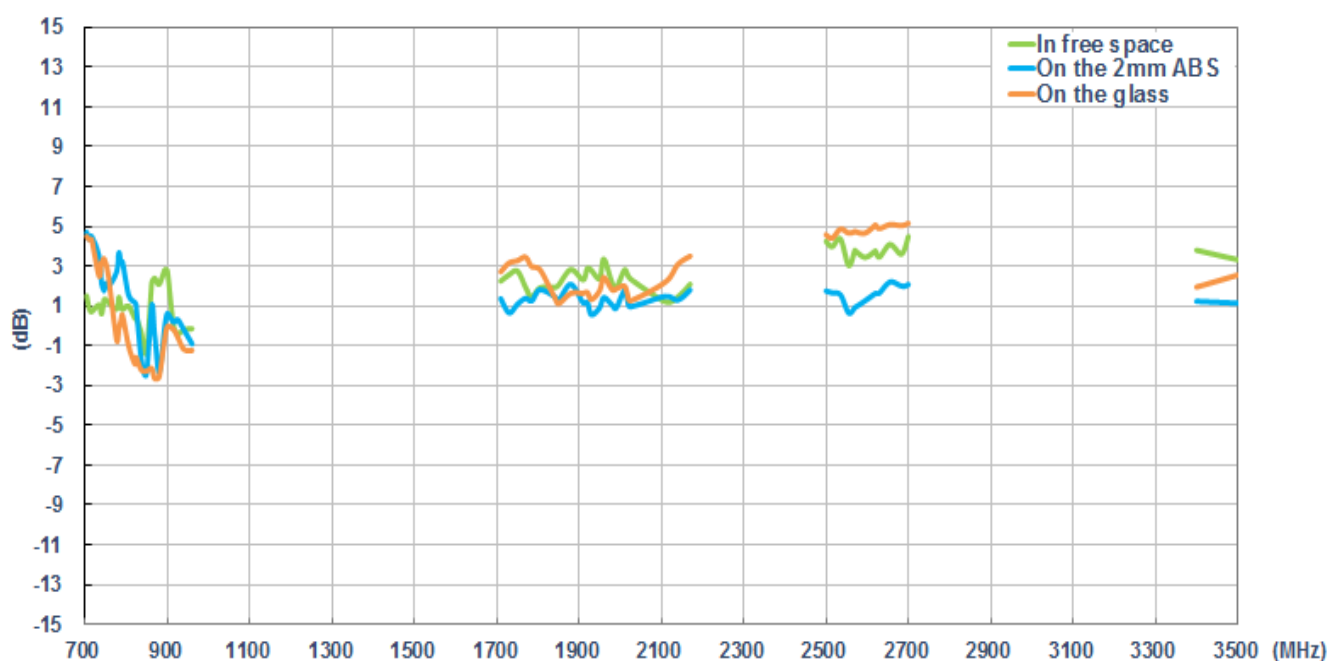
MIMO 1
