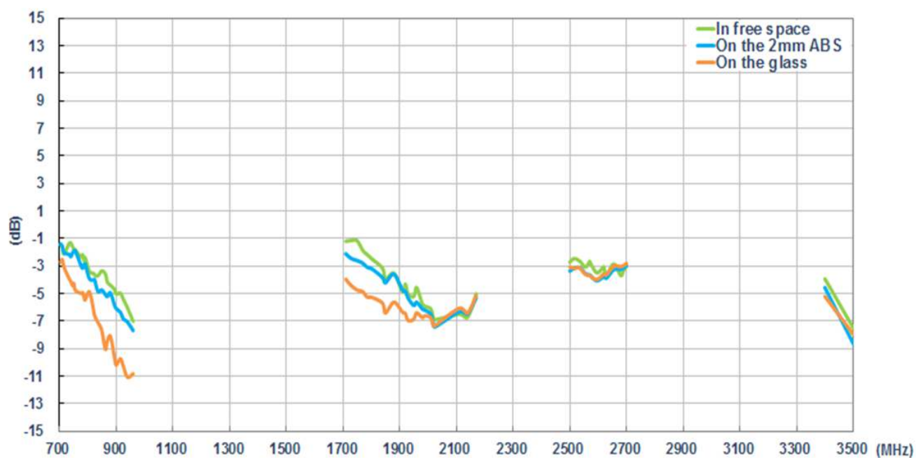
MIMO 2
