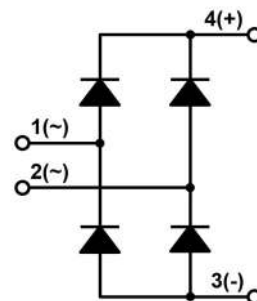
Rectifier Bridge
