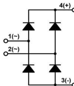
Rectifier Bridge
