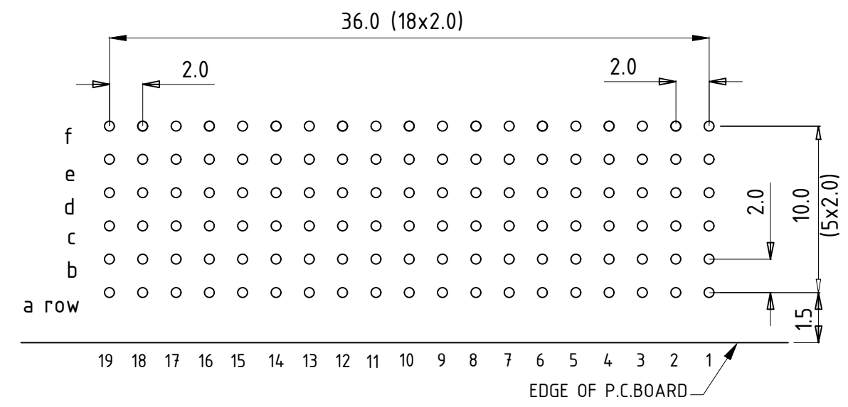
LAY-OUT P.C.B.- HOLE
