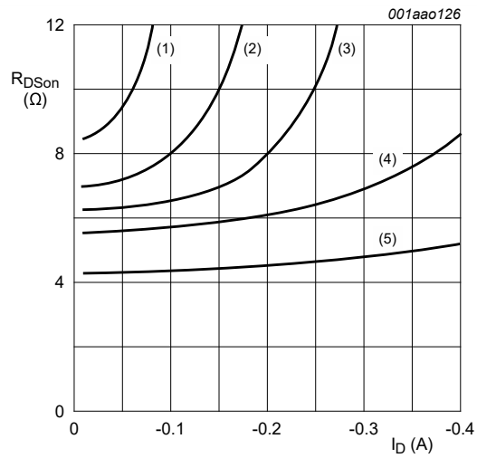
T_j = 25\text{ °C} (1) V_{GS} = -3.0\text{ V} (2) V_{GS} = -3.5\text{ V} (3) V_{GS} = -4.0\text{ V} (4) V_{GS} = -5.0\text{ V} (5) V_{GS} = -10.0\text{ V}
