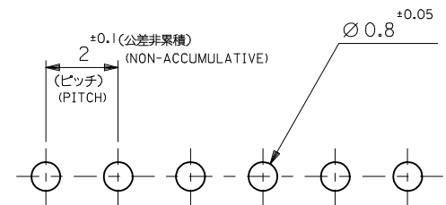
基板取付穴推奨寸法
