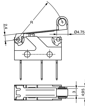
170EL transverse roller
