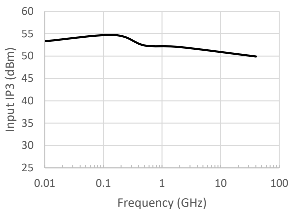
Input IP3 13
