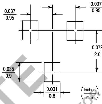
SOT-23
