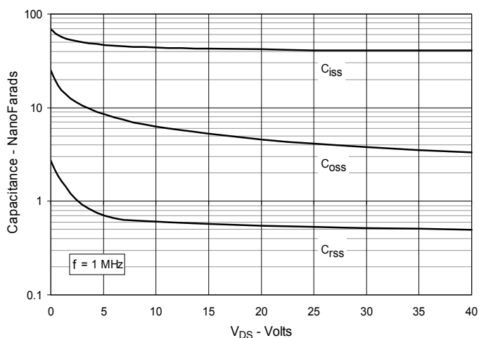
Fig. 10. Capacitance
