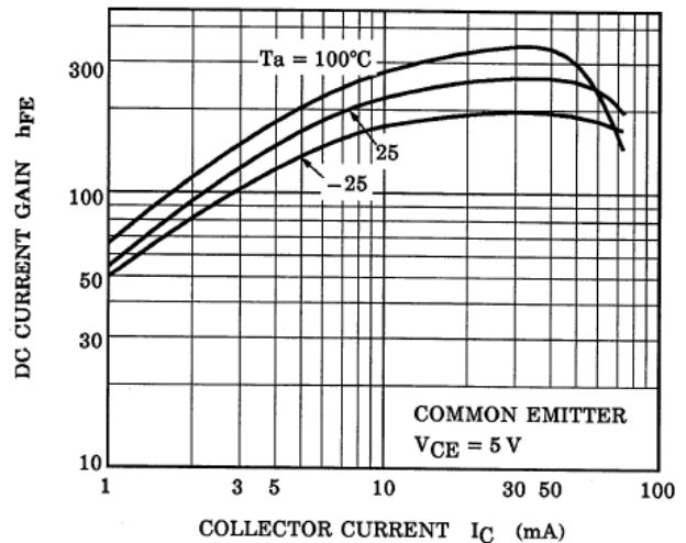
Fig. 10.16 RN1404 h_{FE} - I_C
