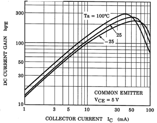
Fig. 10.14 RN1402 h_{FE} - I_C
