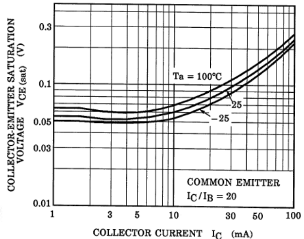
Fig. 10.24 RN1406 V_{CE(sat)} - I_C
