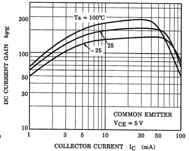
Fig. 10.18 RN1406 h_{FE} - I_C
