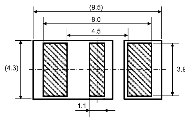
Fig. 10.3.1 (Unit: mm)
