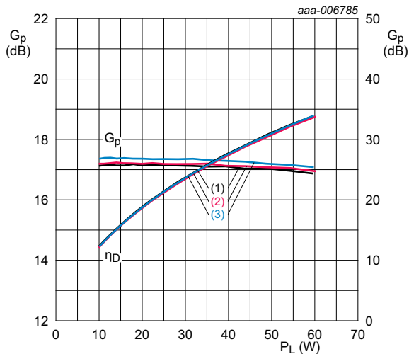
V_{DS} = 28 V; I_{Dq} = 1620 mA. (1) f = 2110 MHz (2) f = 2140 MHz (3) f = 2170 MHz
