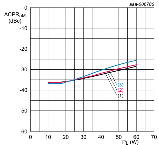
V_{DS} = 28 V; I_{Dq} = 1620 mA. (1) f = 2110 MHz (2) f = 2140 MHz (3) f = 2170 MHz
