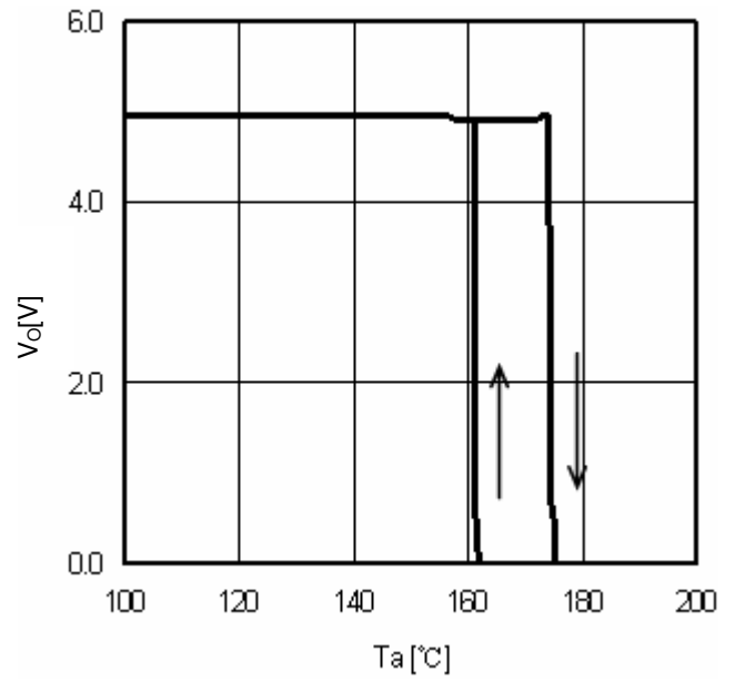
Fig.16 TSD ( I_o=0mA )
