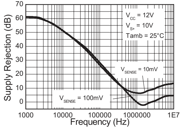
PSRR
