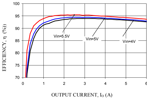
V_o=3.3V
