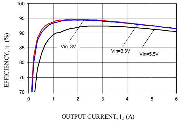
V_o=2.5V
