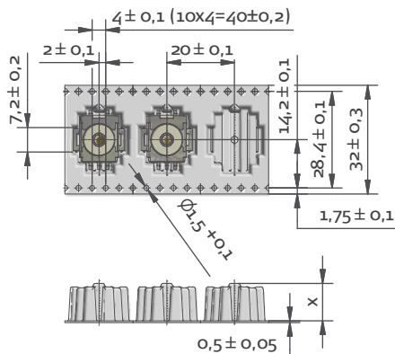
Ende des Gurtes end of tape
