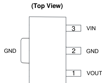
SOT89
