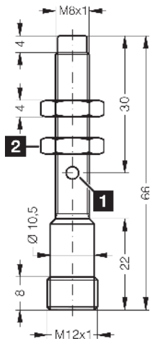
1) LED 2) Schlüsselweite 13 mm BK: schwarz BN: braun BU: blau
