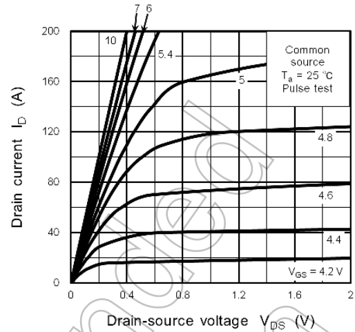
Fig. 9.2 I_D - V_{DS}
