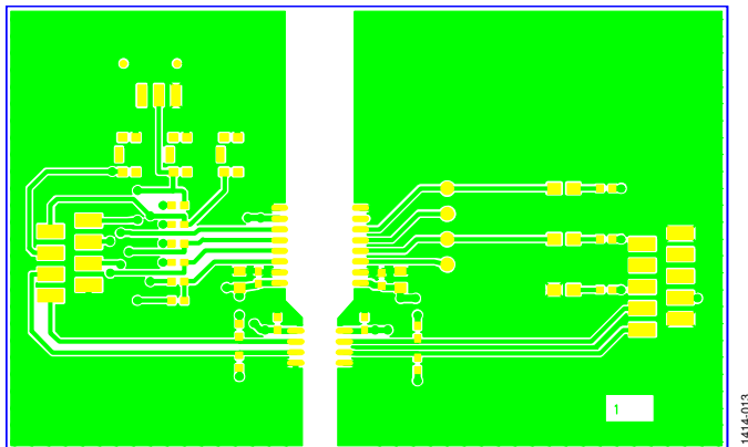
Figure 16. Top Layer
