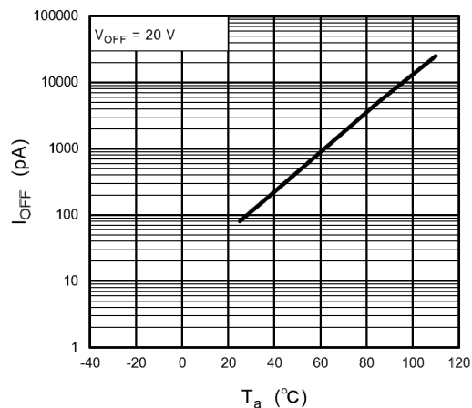
Fig. 12.8 I_{OFF} - T_a
