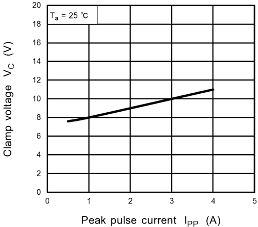
Fig. 5.3.1 V_C - I_{PP}
