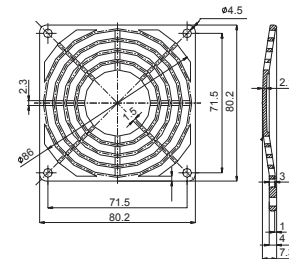
PB-08 For 80mm Fan
