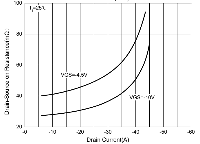
Fig. 4 - R_{DS(ON)} — I_D
