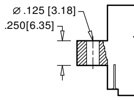
FLUSH MOUNTING (D)
