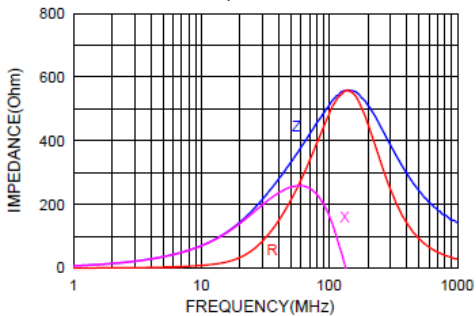
AFBC-Q0402-471
