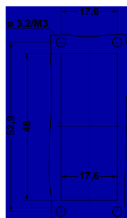
Panel cutout: VS-15-A
