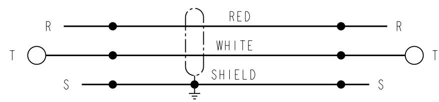
WIRING SCHEMATIC
