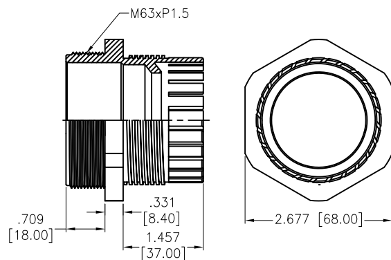
Ⓒ Body
