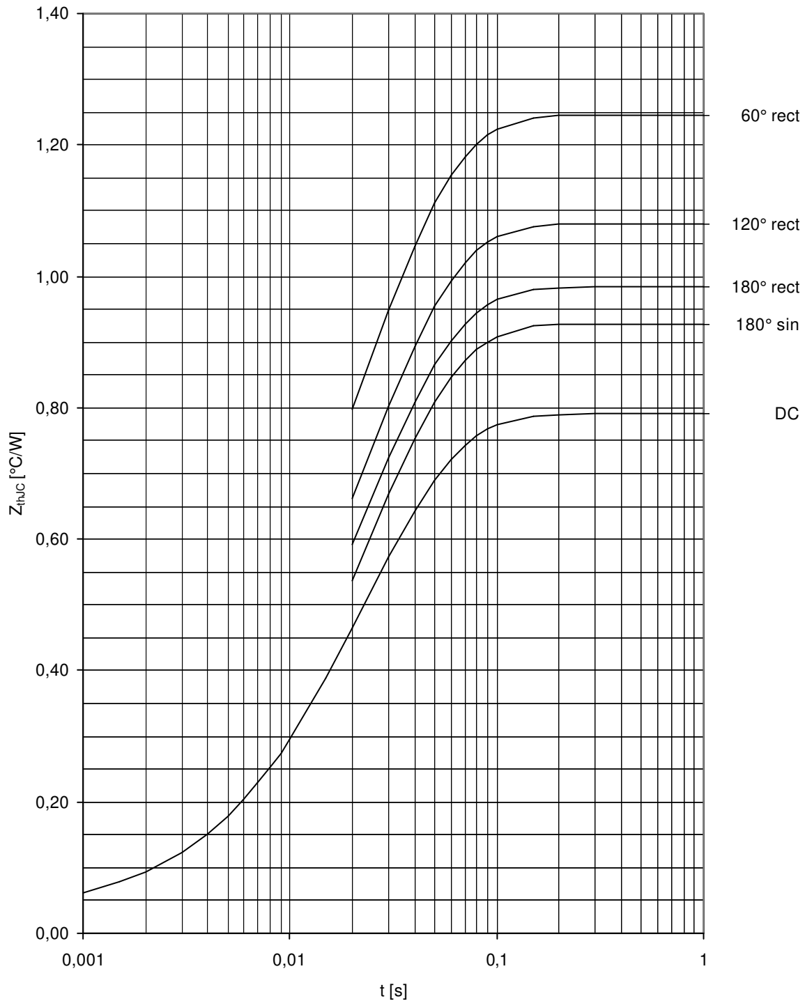
Transienter innerer Wärmewiderstand Gleichrichter / Transient thermal impedance converter Z_{thJC} = f(t) Parameter: Stromflußwinkel / Current conduction angle \theta
