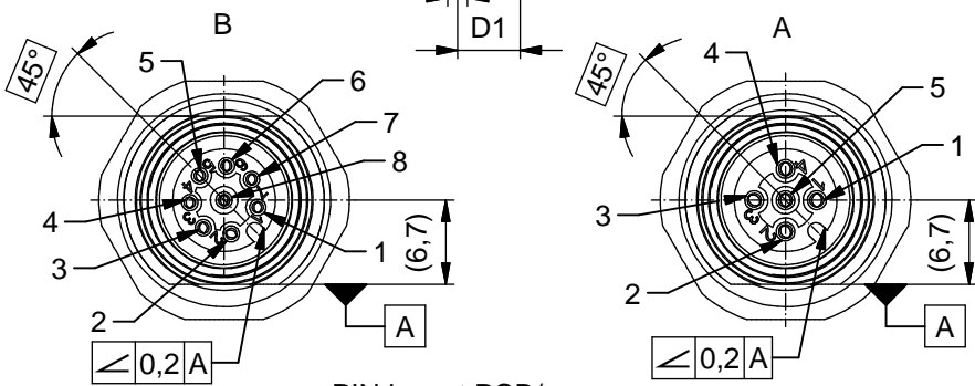
PIN layout PCB/ Lochbild Leiterplatte
