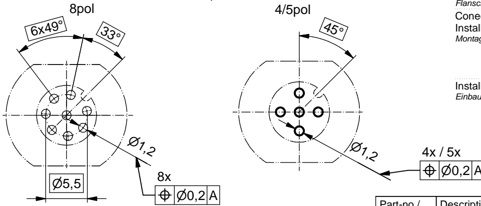
PIN layout PCB/ Lochbild Leiterplatte
