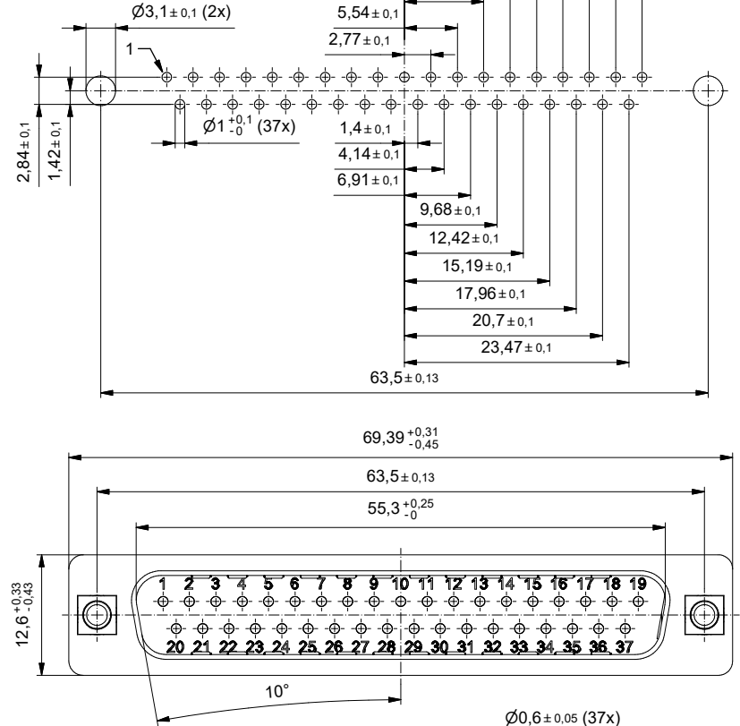
PCB hole drillings (PCB top side) Leiterplattenbohrbild (Leiterplatten Oberseite)
