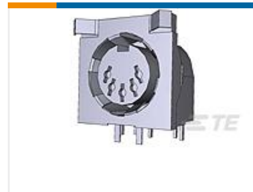
TE Part #5750477-1 5 CIRC DIN RCPT W/GRND FINGERS
