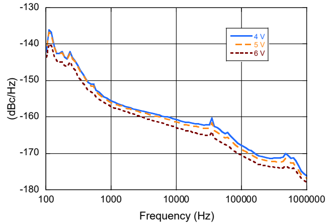
Phase Noise @ 9 GHz, P4dB
