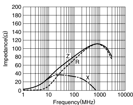
MZA3216S601A
