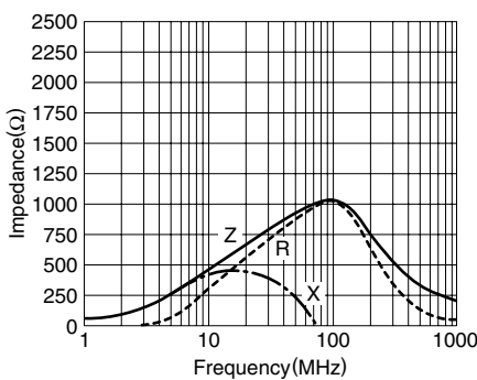
MZA3216S301A
