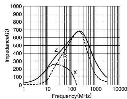
MZA3216S601A
