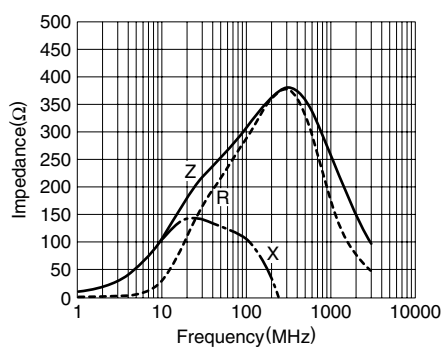
MZA3216S301A
