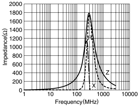
MZA3216D301C
