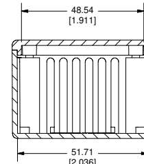
SECTION D-D
