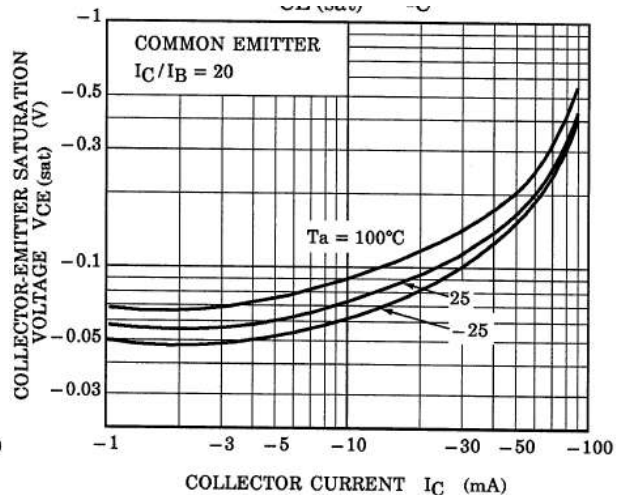
Fig. 10.24 RN2906FE V_{CE(sat)} - I_C
