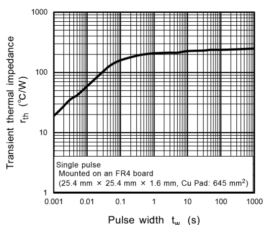
Fig. 8.10 r_{th} - t_w
