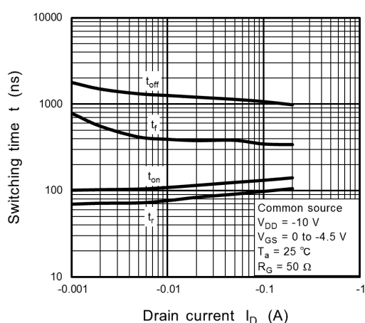
Fig. 8.9 t - I_D
