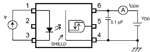
Fig. 12.1.4 I_{DDH} Test Circuit
