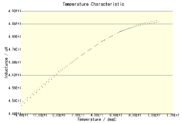
CLF12555T-470M-CA(DC = 0A)
