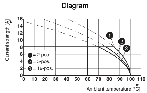
Type: MC 1,5/...-ST(F)-3,5 AU with MCV 1,5/...-G(F)-3,5 AU
