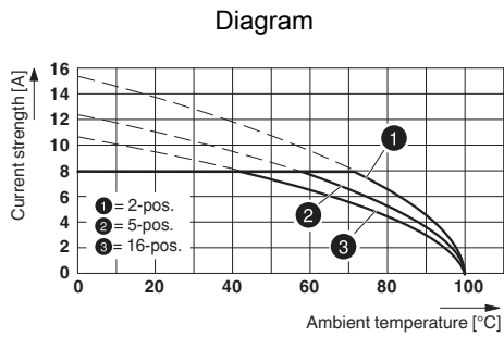
Type: MCVR 1,5/...-ST-3,5 AU with MCV 1,5/...-G-3,5 AU
